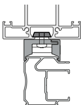
Afstandsplaat voor tweede geleiderzijde bij montage met zijbevestiging of montageverlengstuk
