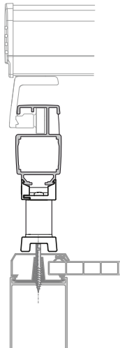
Montagevoet (verschillende hoogtes)
