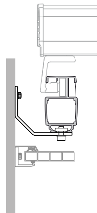
Zijbevestiging wand
