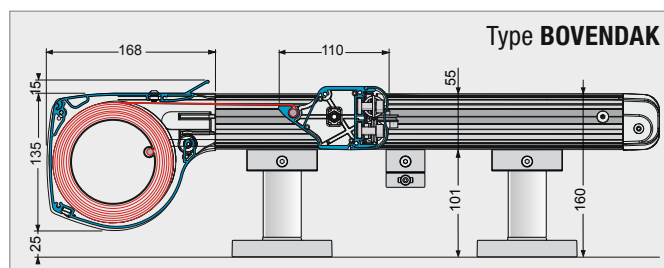
Dubbele steun met drukplaat voor montage op glazen dak Murano
