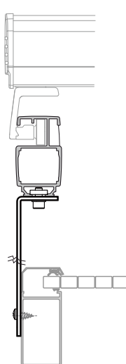
Zijbevestiging
