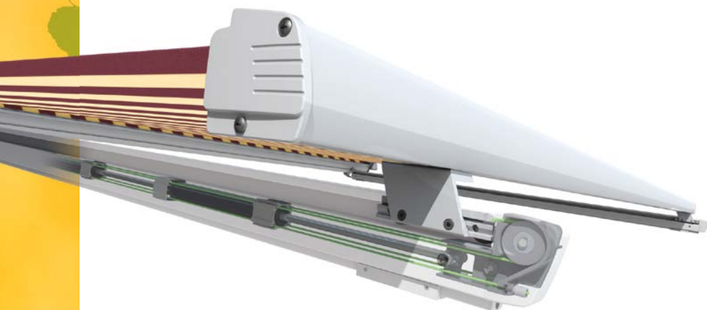
Voorlijst met geleiding met naaldlagers
