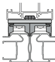
Dubbele steun met drukplaat voor montage op glazen dak Murano
