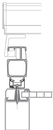
Railhouder (standaard)
