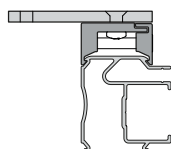
Montageverlengstuk
