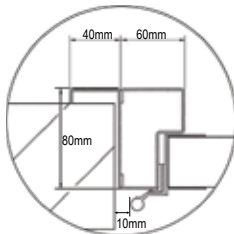
Profielafmeting
