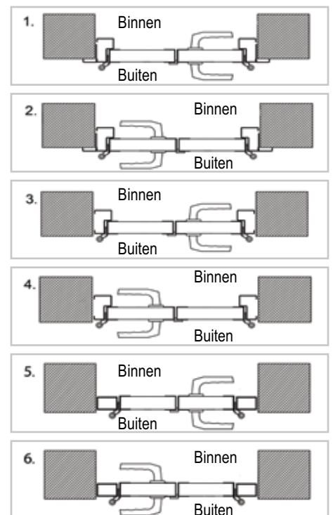
Inbouwvarianten
